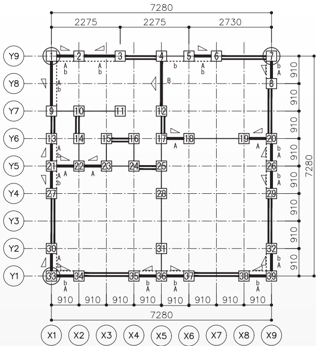
耐力壁図と集計表の整合
